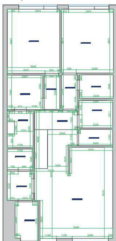
Обмерный план
