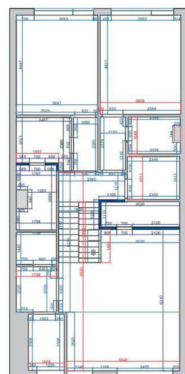
Обмерный план после перепланировки
